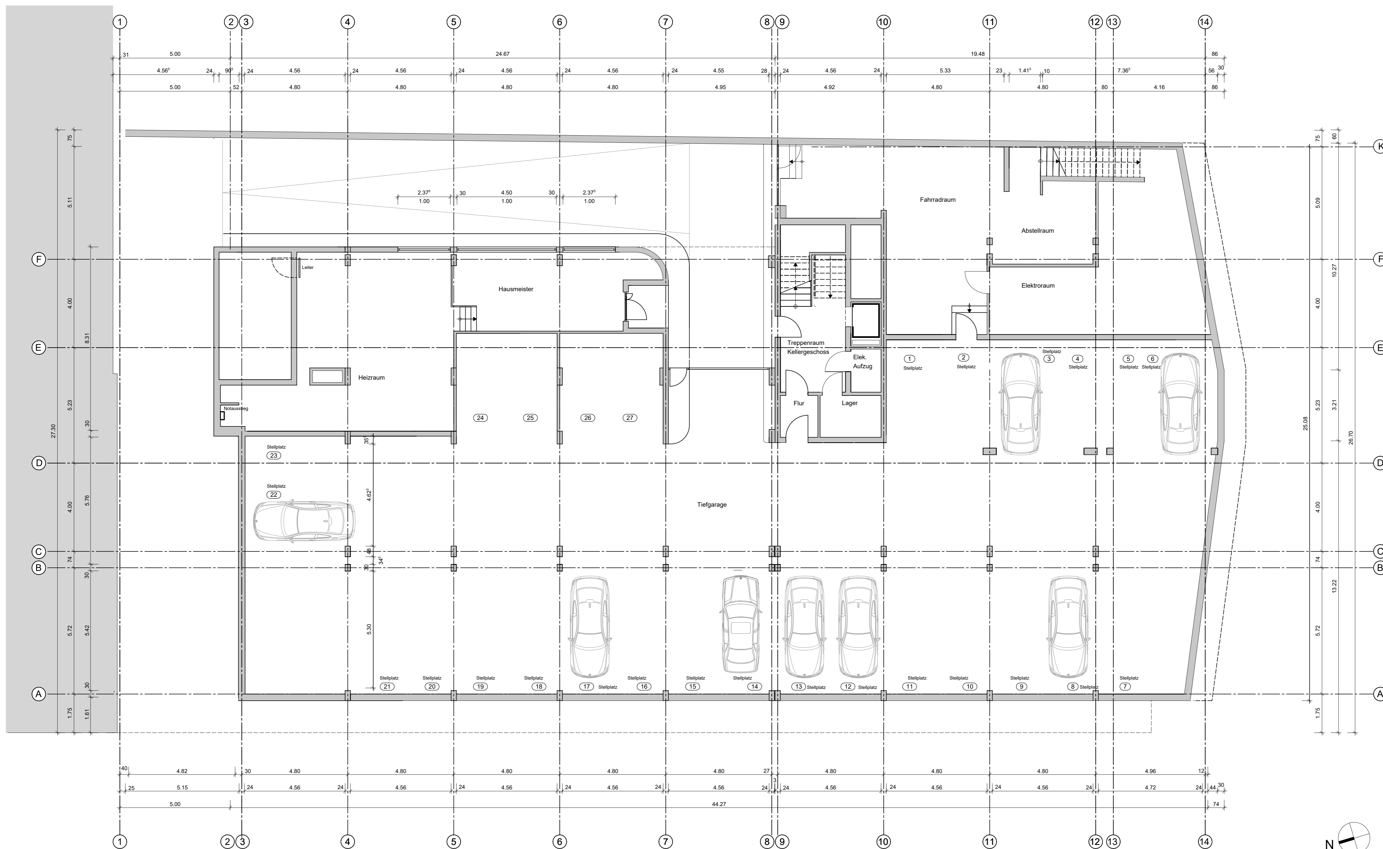
KELLERGESCHOSS
