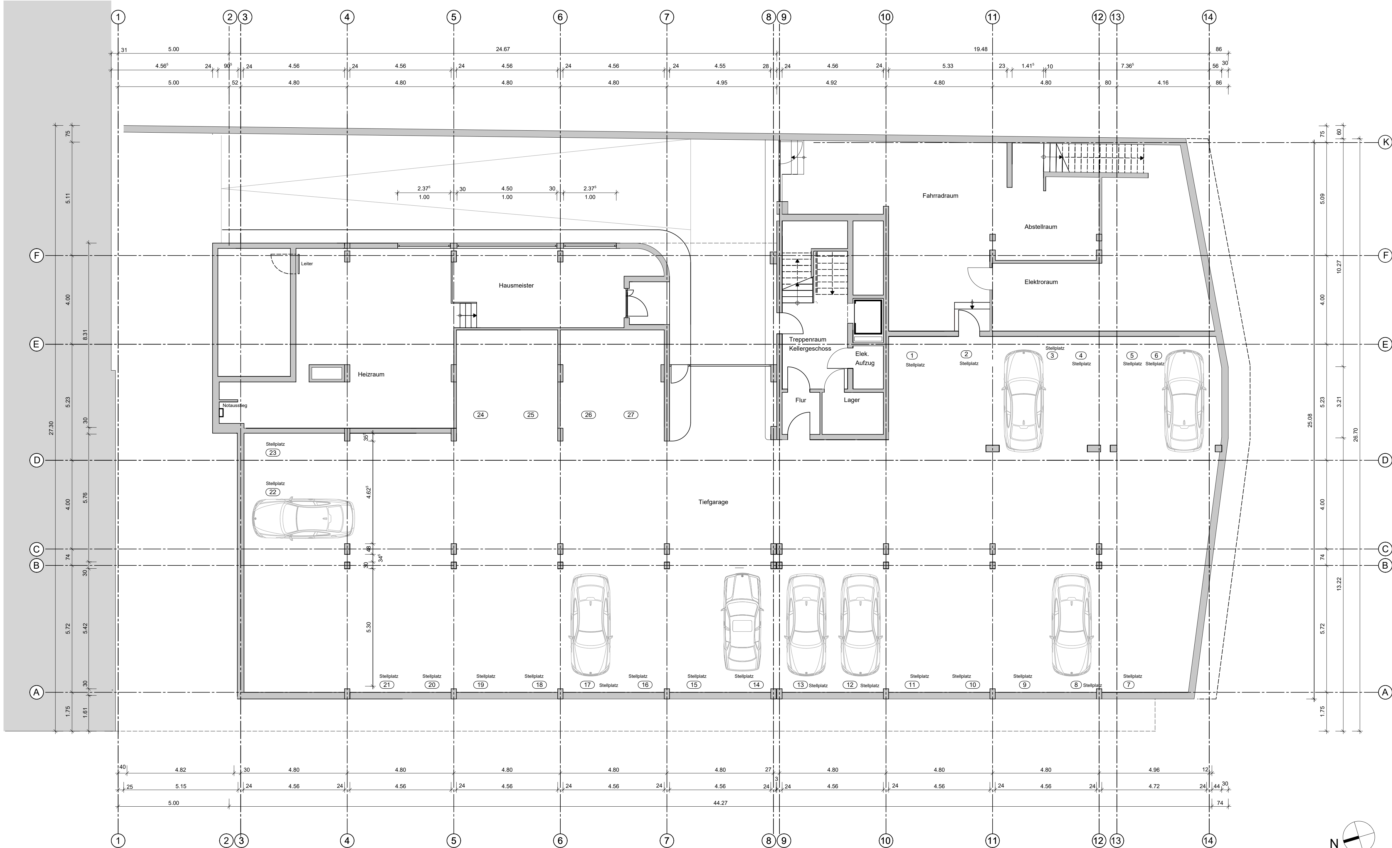
KELLERGECHOSS
