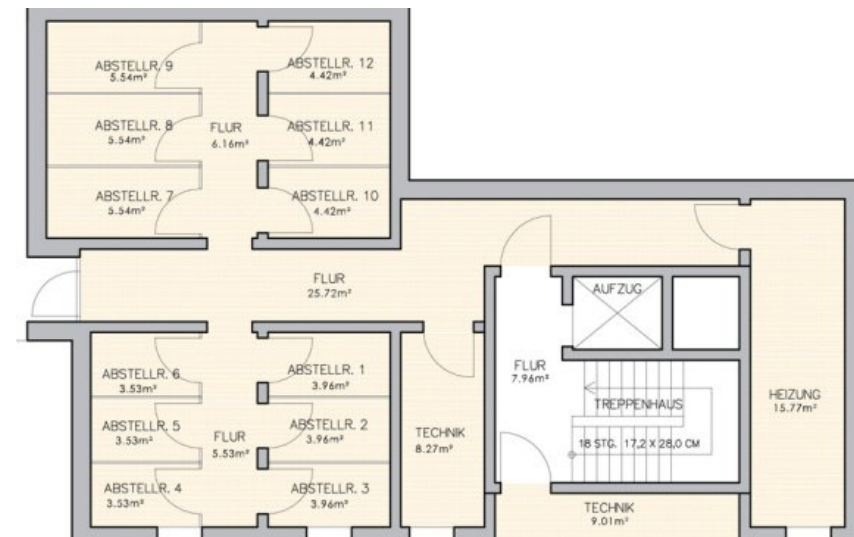
Kellergeschoss Grundriss
