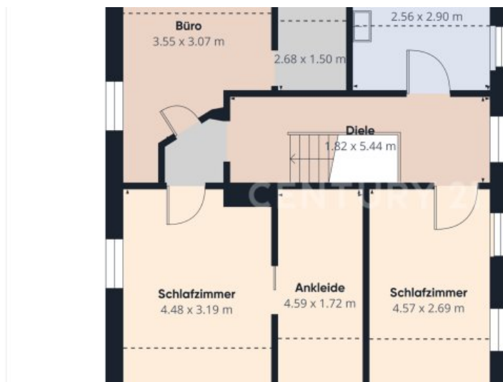
Grundriss 1.OG
