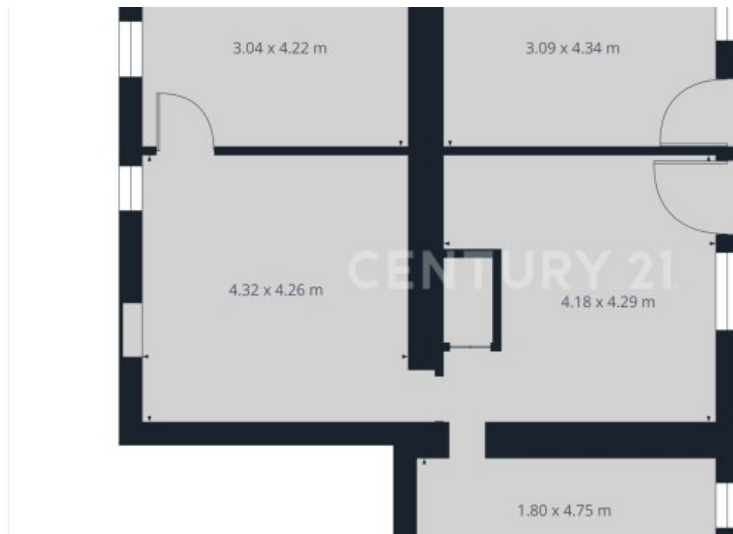
Grundriss Keller
