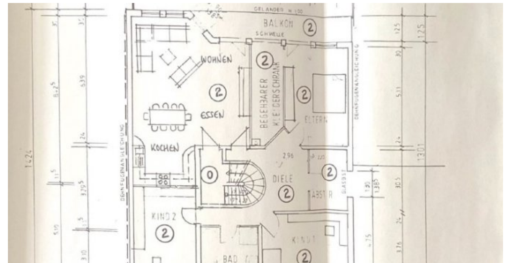
Grundriss OG
