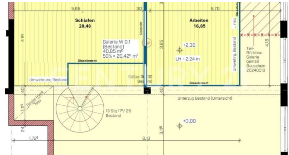
Grundriss Galerie mit 2 Schlafzimmern als 3ZKB
