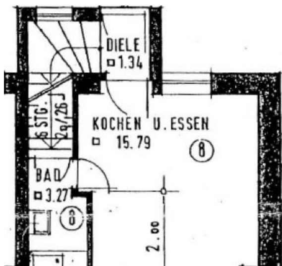
Grundriss Erdgeschoss
