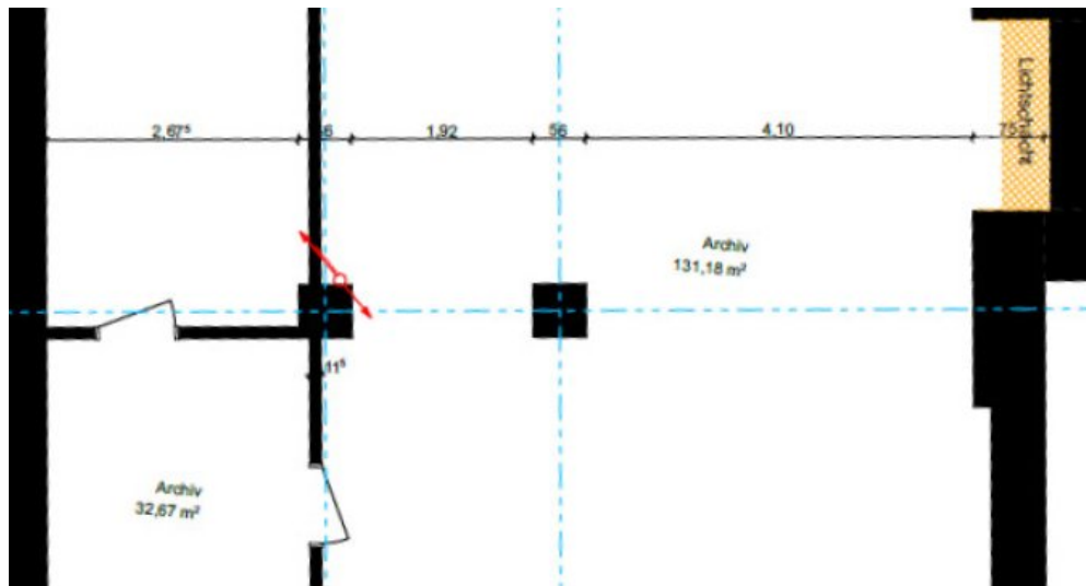
Grundriss A 1
