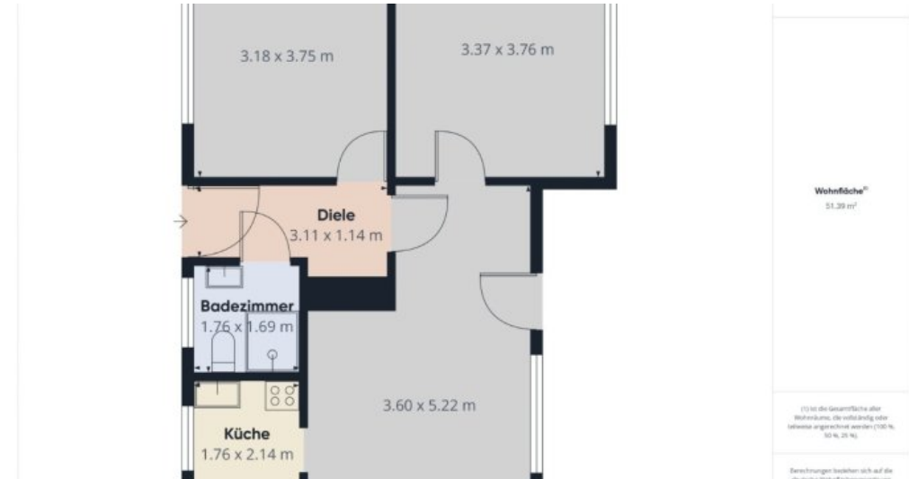
Grundriss
