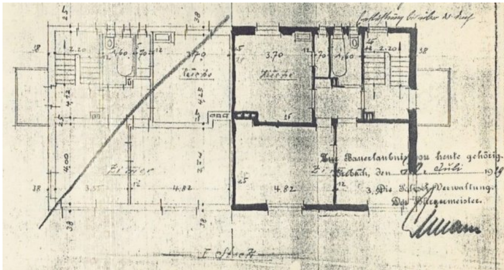
Grundriss OG 1
