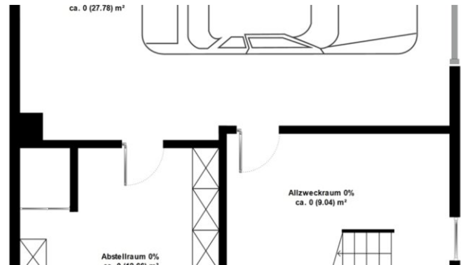
Grundriss KG
