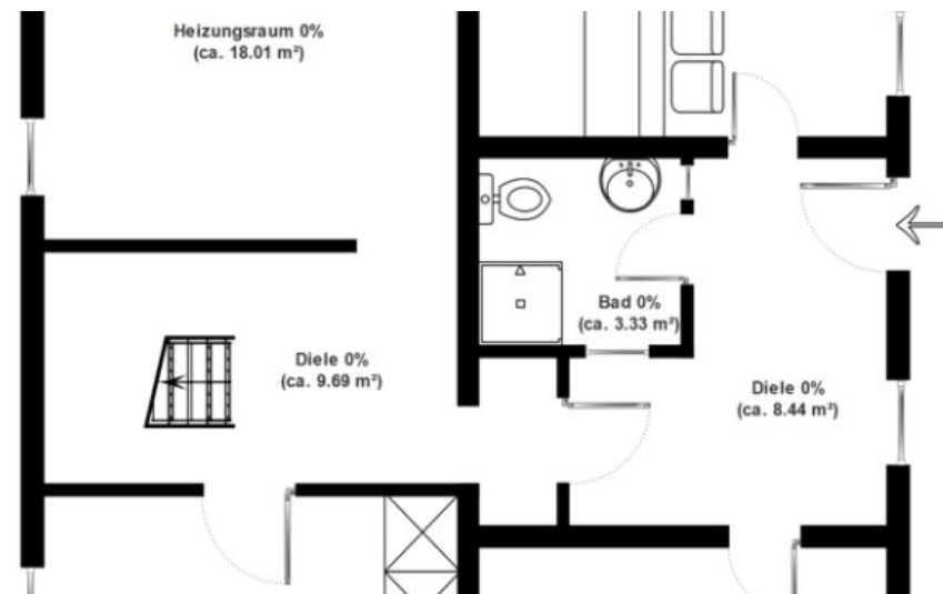
Grundriss KG
