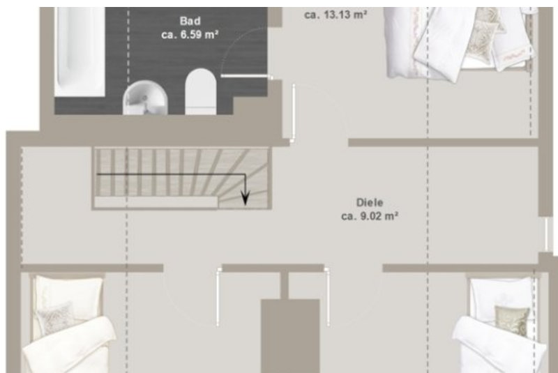
Grundriss DG
