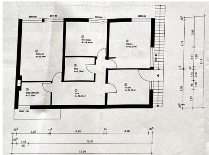
Grundriss WHG 2
