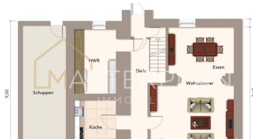
Grundriss EG
