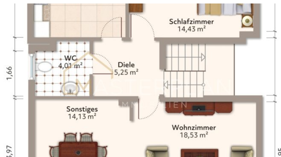
Obergeschoss
