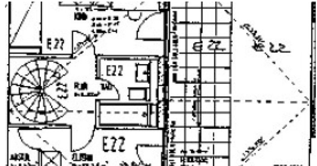
Grundriss 2.OG
