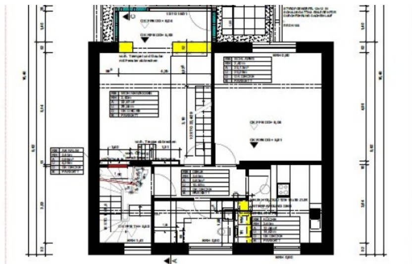
Grundriss DG
