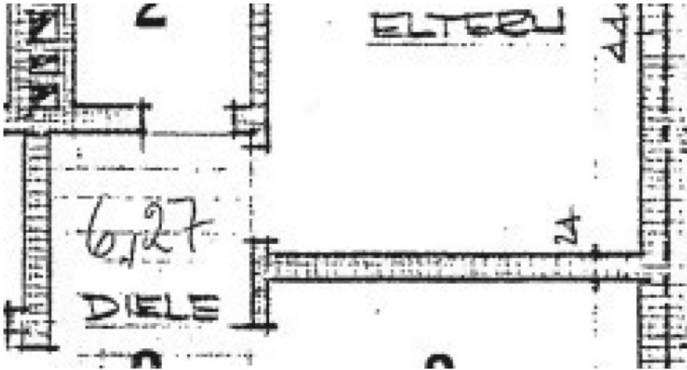
Grundriss EG rechts
